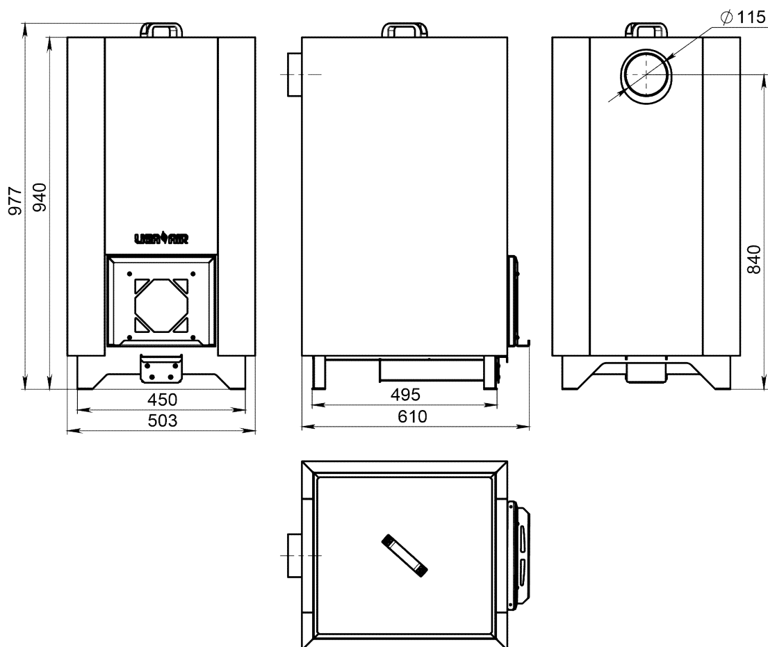
Рисунок-2. Габаритно-присоединительные размеры
